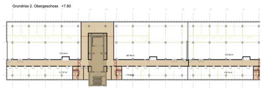
Abb. oben: Grundriss NanoelektronikZentrumDresden Quelle: IPRO
