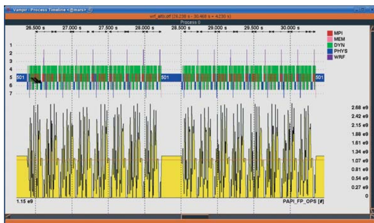
Vampir Screenshot: Zeitlinie eines einzelnen Prozesses mit Hardware Performance Counter
